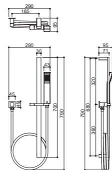
Ref. RB81510 Acabamento rose gold [5091]. Flexível de metal de 1,5 metros. Ducha de barra para box e banheira com regulagem. Vazão: 8 l/min com 15 m.c.a. Pressão recomendada: de 15 m.c.a. até 40 m.c.a.
