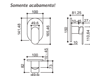
Ponteira de metal. Cartucho ø45mm
